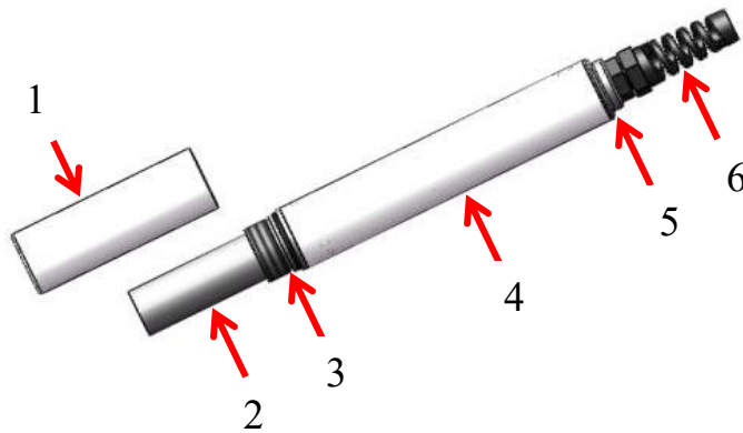
图 2.1 SD-14A16 型 pH 数字传感器
